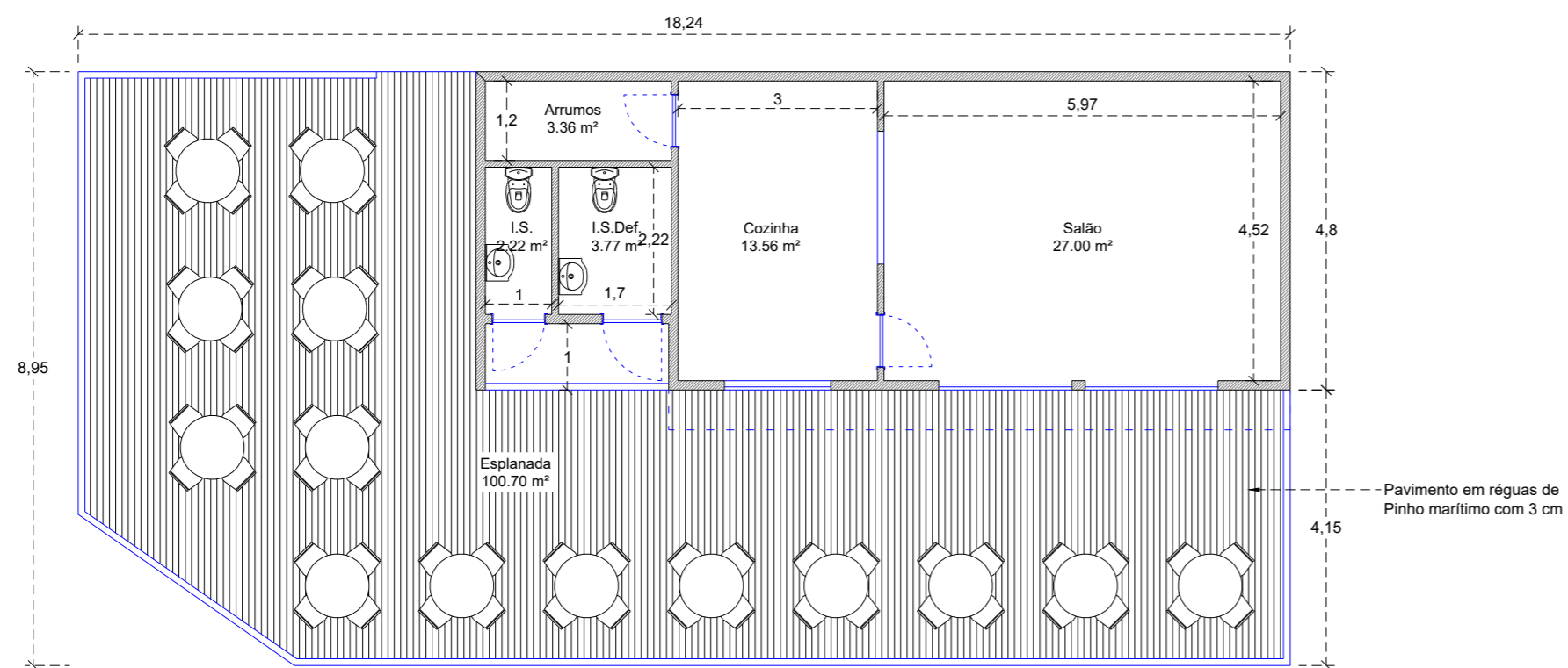
PLANTA DO RÉS-DO-CHÃO
