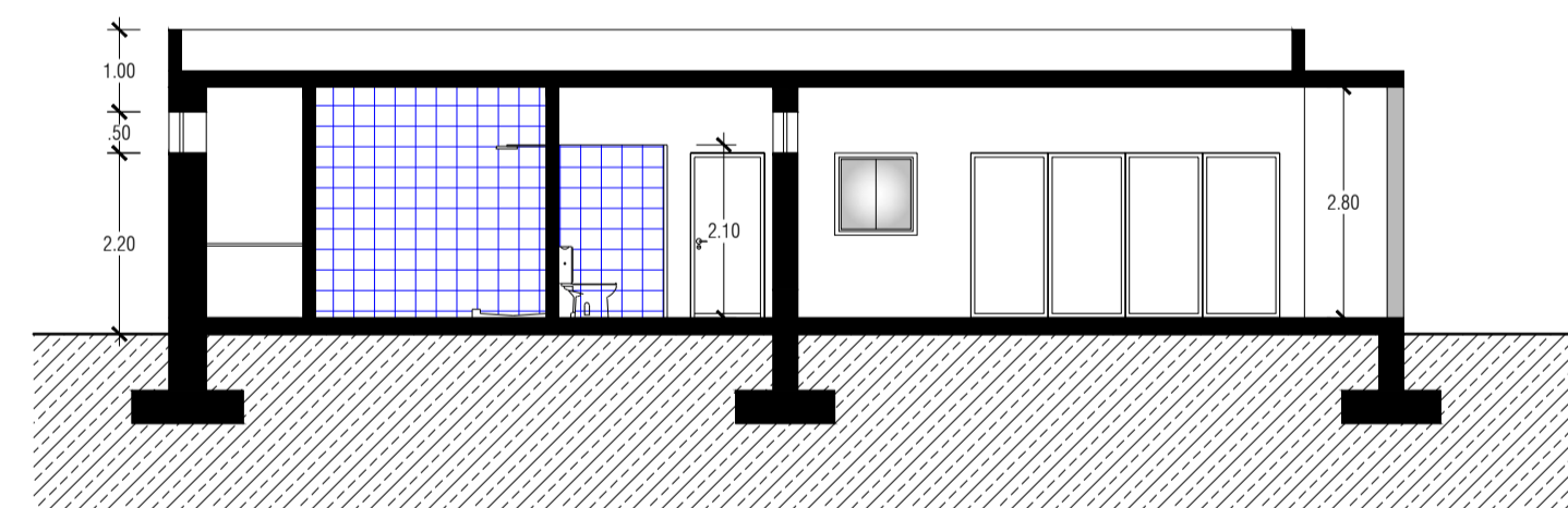
CORTE AA'
