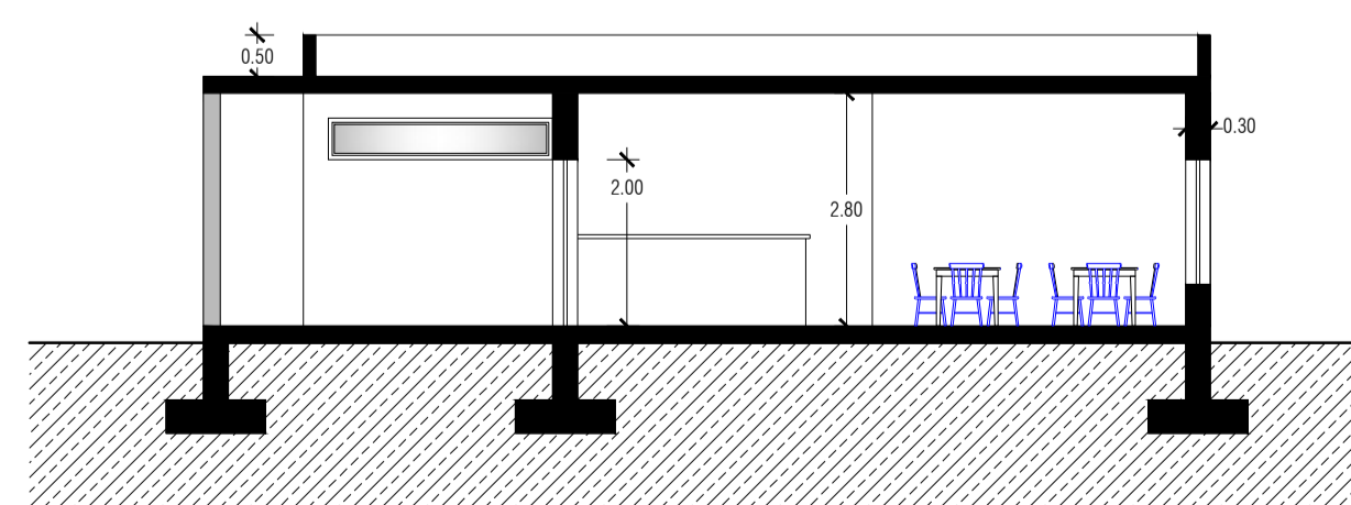
CORTE BB'
