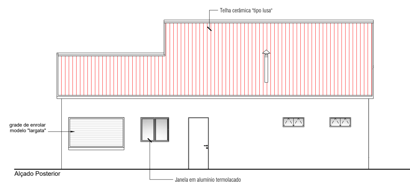
Alçado Posterior
