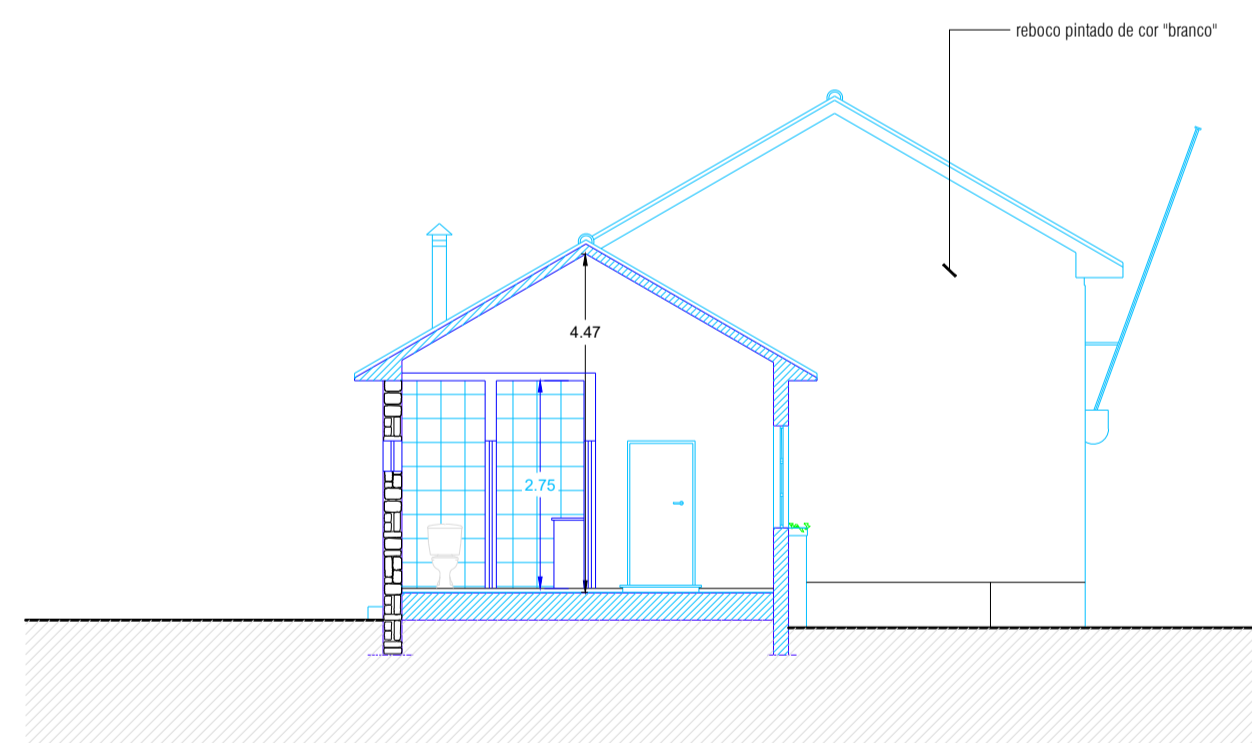
Corte AA'
